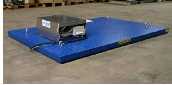
Flachformhebetisch, 2040 mm x 1400 mm, Nutzhub 700 mm, Nutzlast 1000 kg, Bauhöhe 100 mm
